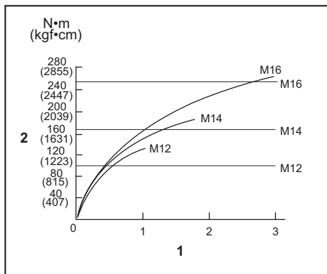
1. Χρόνος στερέωσης (δευτερόλεπτο) 2. Ροπή στερέωσης
