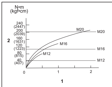
1. Χρόνος στερέωσης (δευτερόλεπτο) 2. Ροπή στερέωσης
