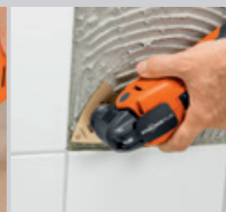
De hardmetalen schraper maakt tegelijk glad en zorgt voor een vlakke ondergrond.
